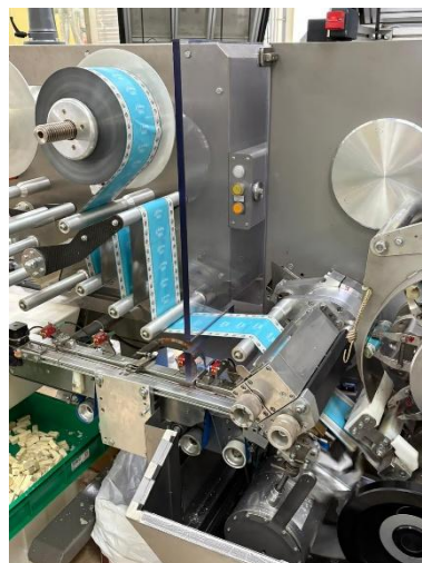
Une emballeuse
